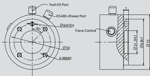
AUBO-i3 Tool End Flange
