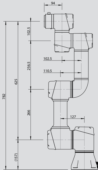
AUBO-i3 Dimensions
